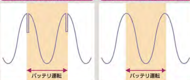
ラインインタラクティブ方式の出力波形 常時インバータ給電方式の出力波形
